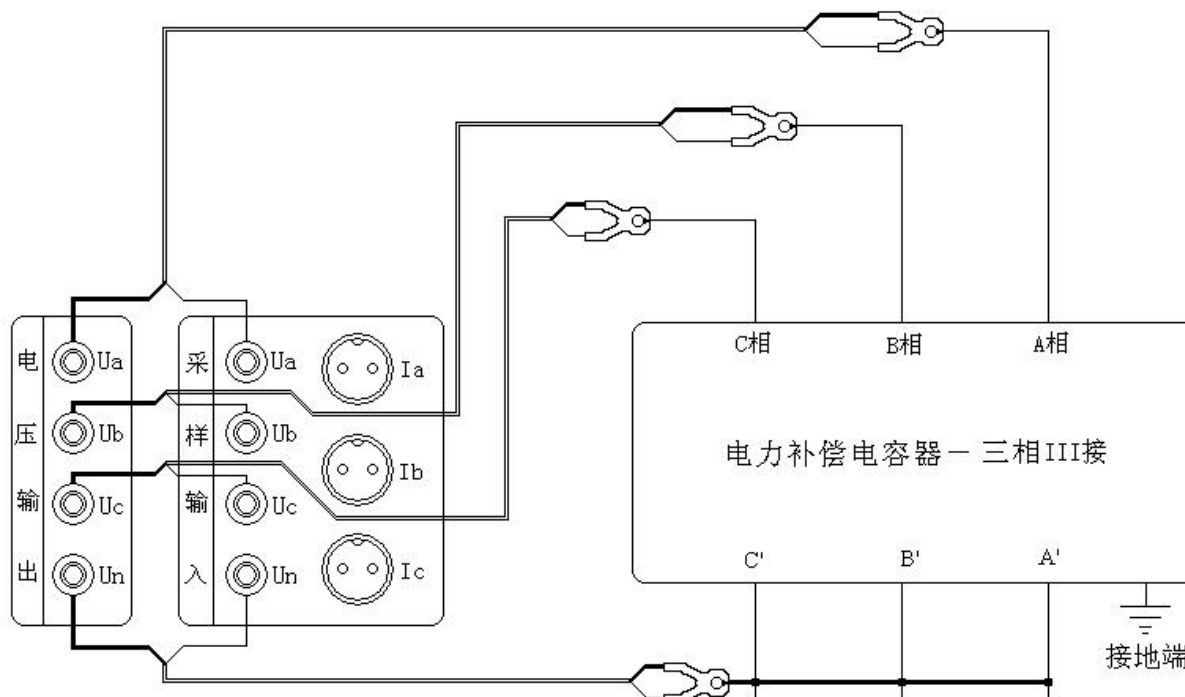
图 24、三相 III 接电容内部互感器测试接线
