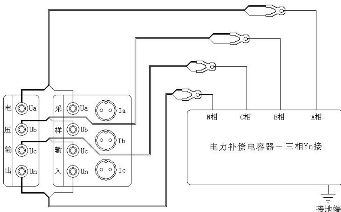
图 22、三相 Yn 接电容内部互感器测试接线
