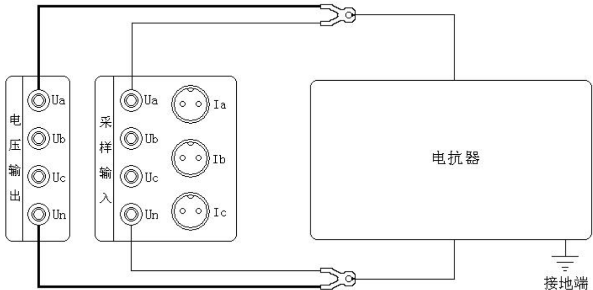
图 25、单相电感测试接线
