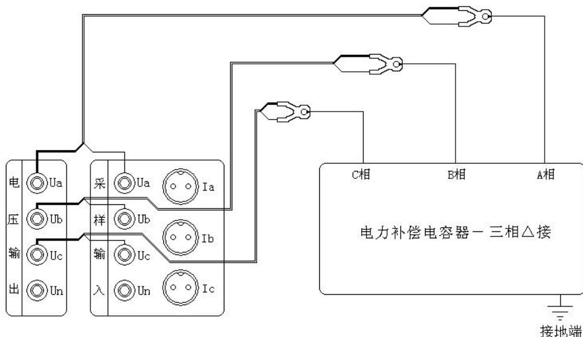
图 23、三相 \Delta 接电容内部互感器测试接线
