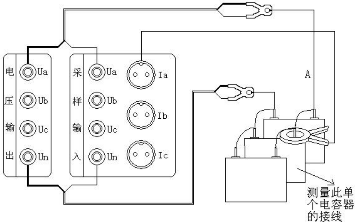
图 19、并联电容组单只电容测试接线
