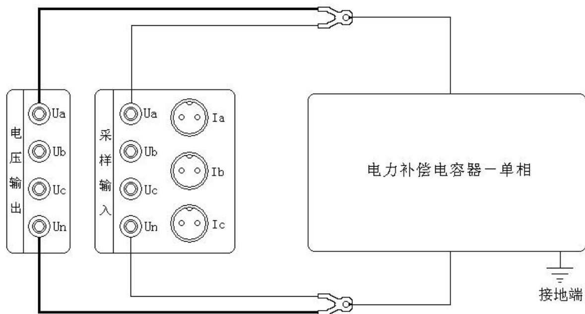
图 20、单相电容内部互感器测试接线
