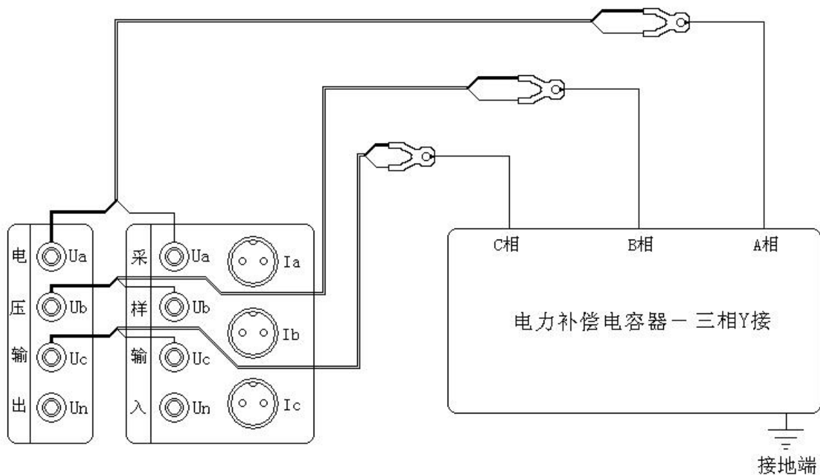
图 21、三相 Y 接电容内部互感器测试接线
