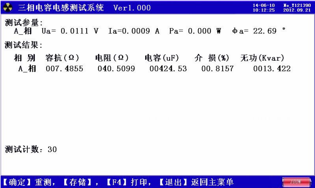
图 14、单相电容测试结果界面
